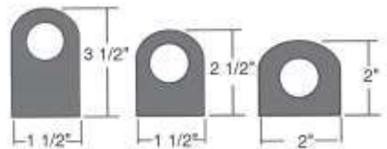
Stabilisator-Rahmen-Buchsen
